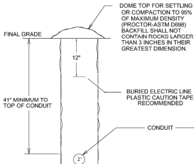
CONDUIT INSTALLATION
